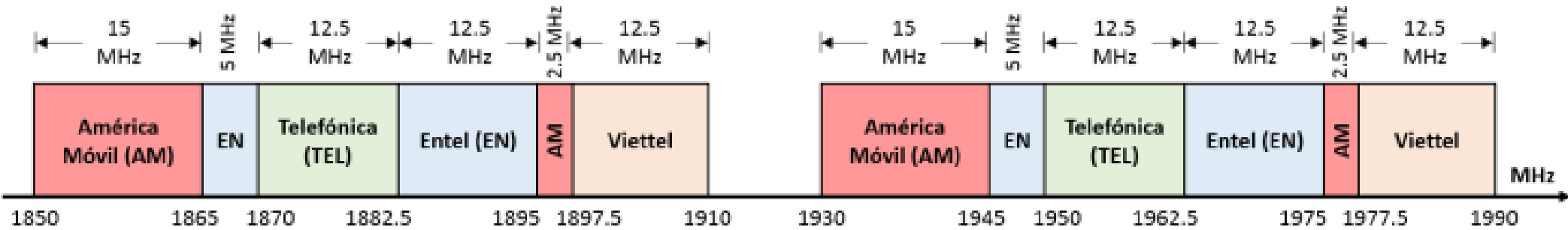
Figura N° 66.- Banda de 1900 MHz
