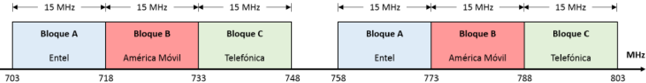
Figura N° 62.- Banda de 700 MHz
